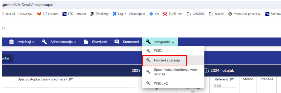
Slika 1 - Preuzimanje projekta
