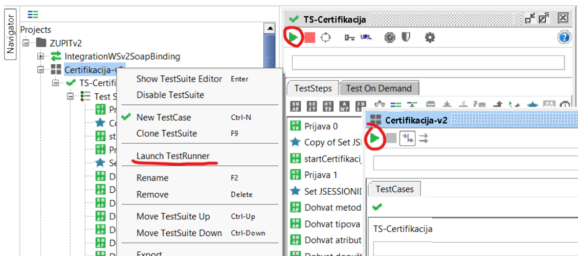
Slika 4 - Načini pokretanja
