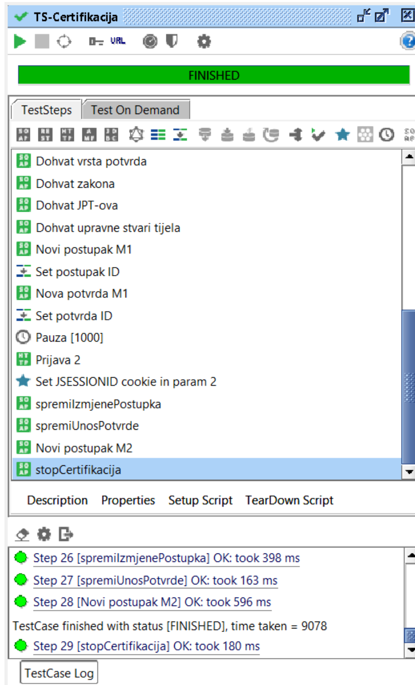
Slika 5 - Uspješno pokretanje
